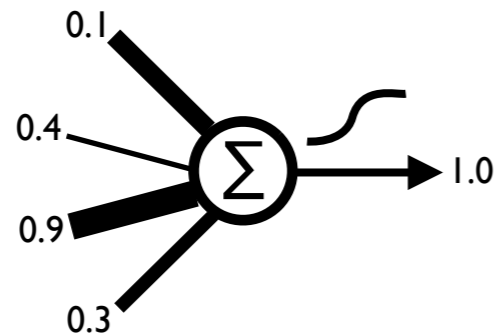
Perceptron
